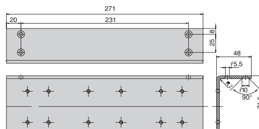
Угловая монтажная пластина DC130
