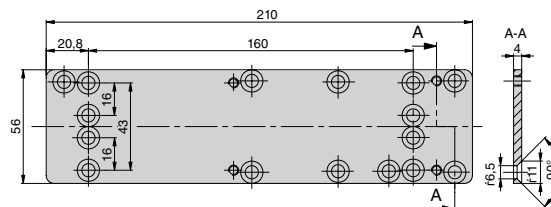
Прямая монтажная пластина DC130
